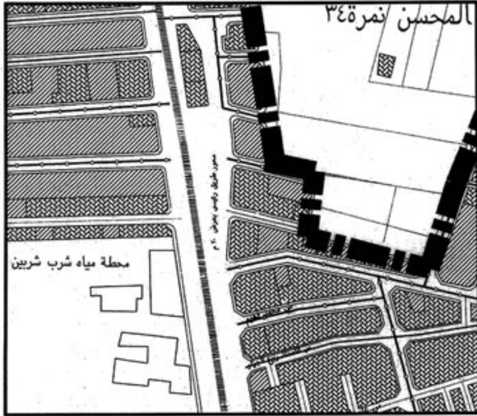
المخطط التفصيلي لمنطقة محطة مياه الشرب - مدينة شربين
