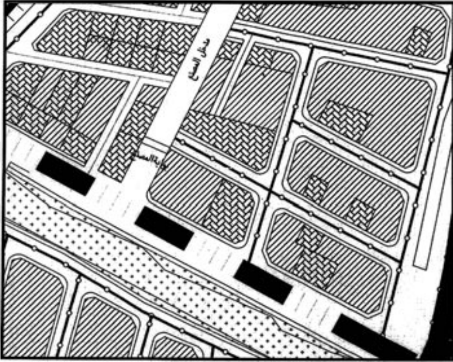
المخطط التفصيلي لمنطقة تقسيم رمضان السلاب و الإسكان الحكومي - مدينة شربين
