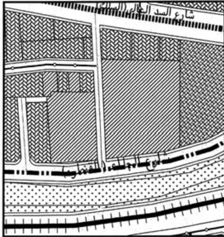
المخطط التفصيلي لمنطقة تقسيم رمضان السلاب و الإسكان الحكومي - مدينة شربين
